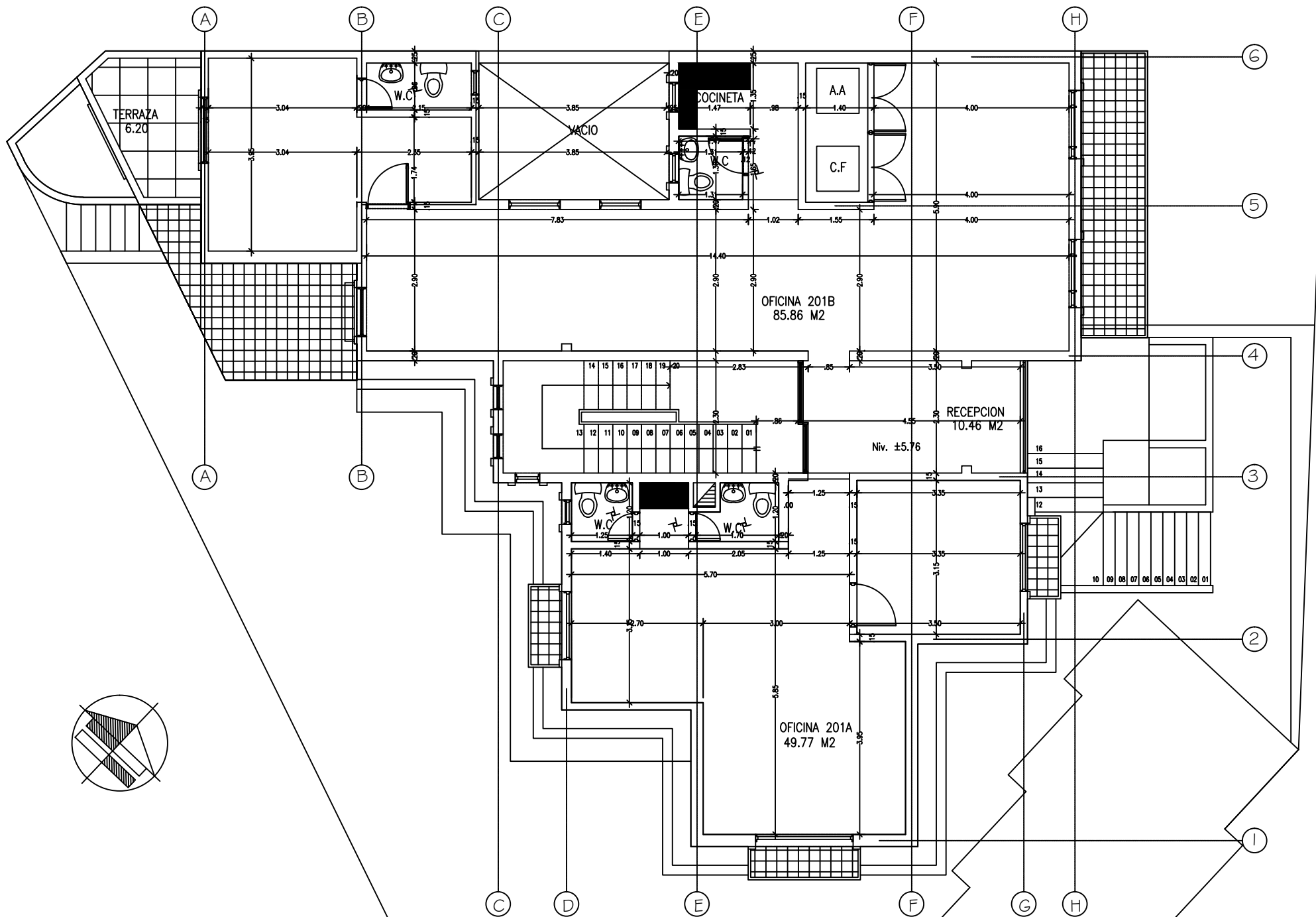
PLANTA SEGUNDO PISO
